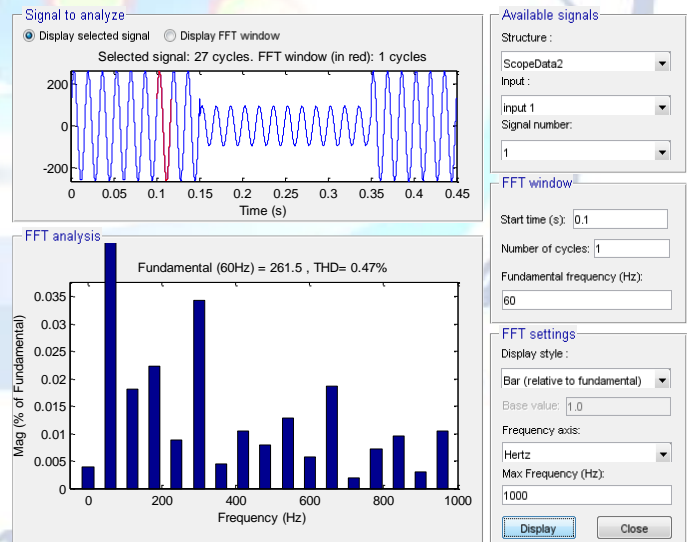
Input THD
